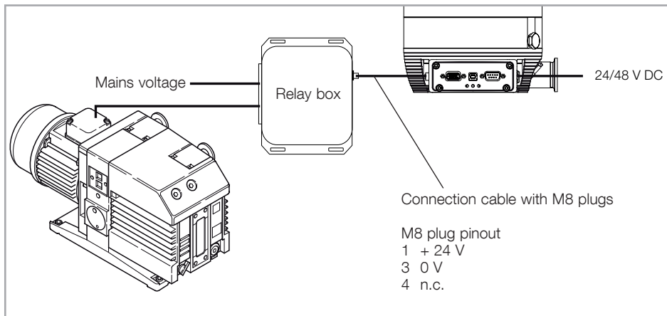
Fig. 3 Wiring diagram
