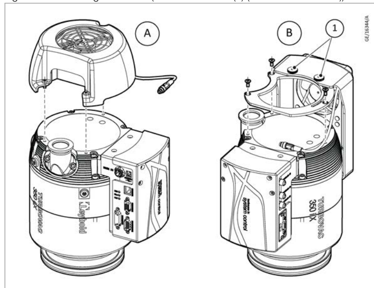
A. Axial air cooler
